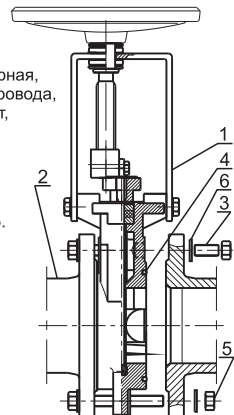
Схема монтажа
